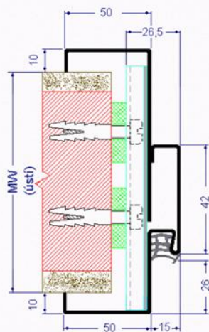
DZbTG - dělené zárubně s drážkou pro těsnění pro dveře s polodrážkou
