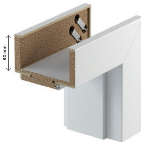
Průřez zárubně
