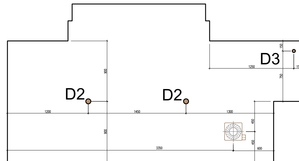
POZICE A TYP SVĚTEL + ELEKTRO:
